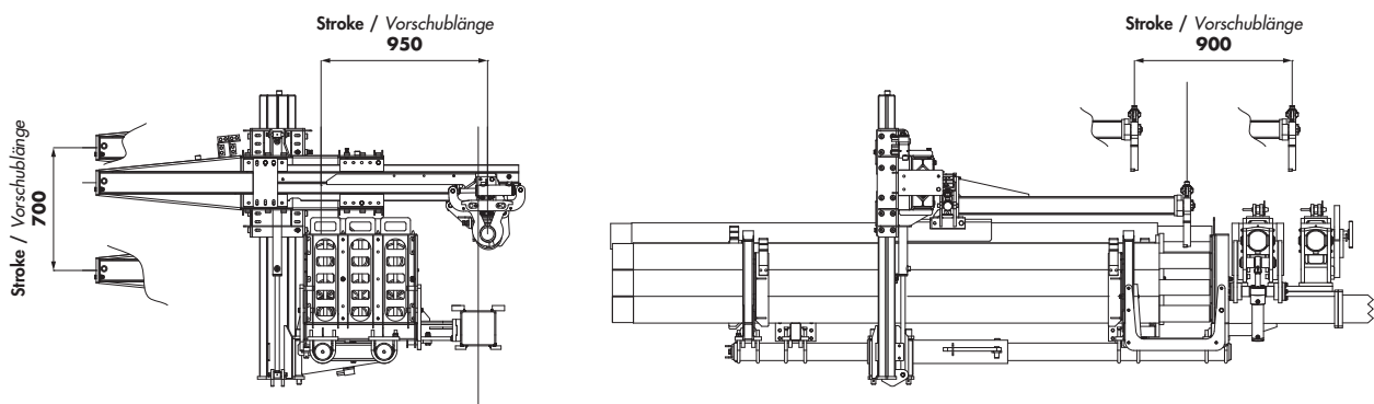
Rods / Innenrohr
